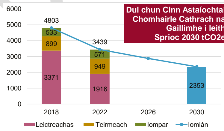
Fíor 2-5 Dul chun Cinn astaíochtaí iomlána Chomhairle Cathrach na Gaillimhe i leith tCO 2 e Sprioc 2030
