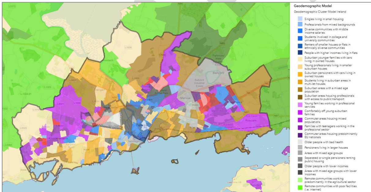
Fíor 4-6 Teasláráid déine geodhéimeagrafaí limistéar riaracháin Chomhairle Cathrach na Gaillimhe
