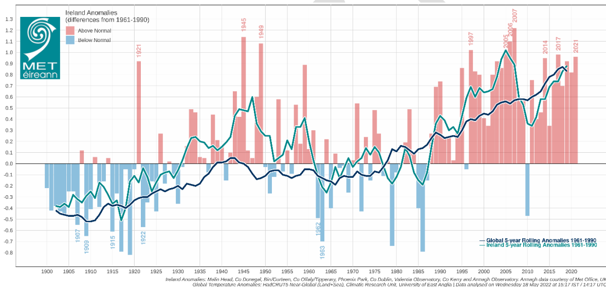
Fíor 1-1 Meánteocht Bhlíantúil Aer Dromchla (1900-2021) d'Éirinn ina léirítear méadú thart ar 0.9°C le 120 bliain anuas, Foinse: Met Éireann, an Creat Aeráide Náisiúnta do Sheirbhísí Aeráide (NFCS)
