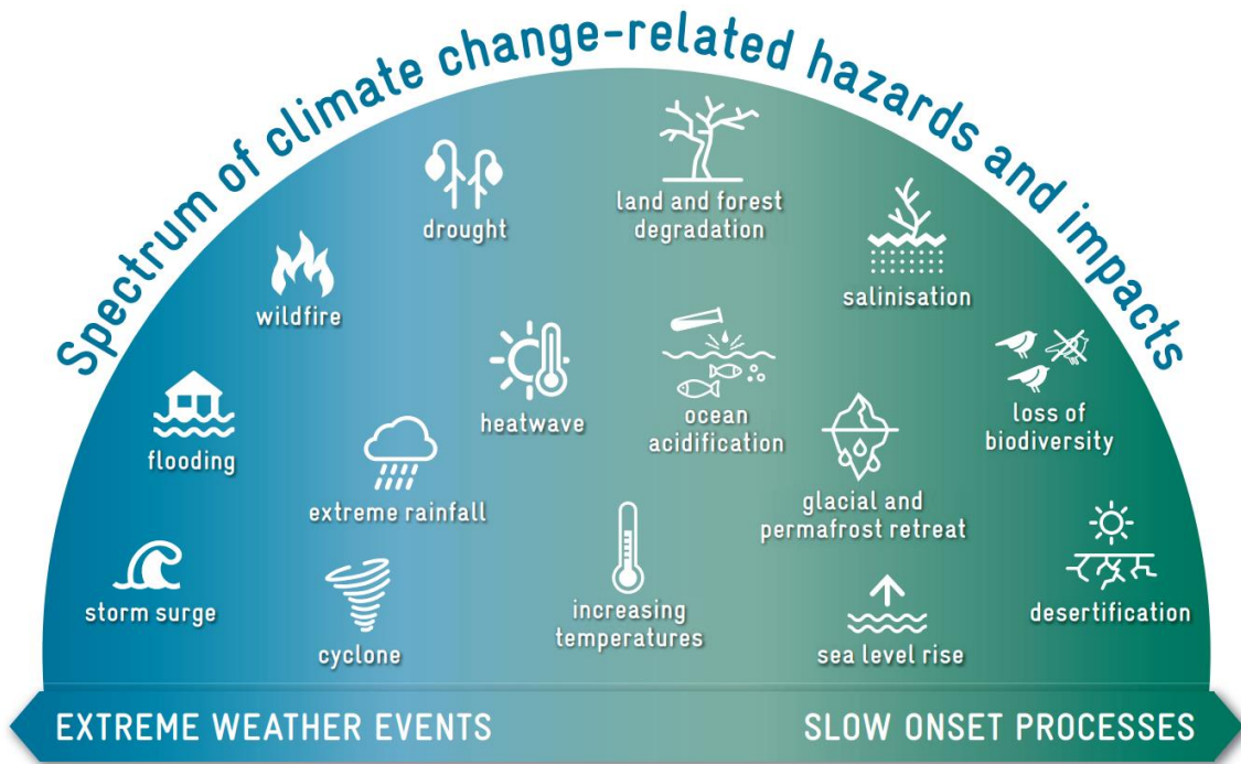
Fíor 1-2 Réamh-mheastacháin Fhéideartha Aeráide Amach Anseo d'Éirinn (Foinse: Bunaithe ar: ©GIZ/an Clár Domhanda um Measúnú agus Bainistiú Riosca d'Oiriúnú d'Athrú Aeráide (Caillteanas agus Díobháil)
