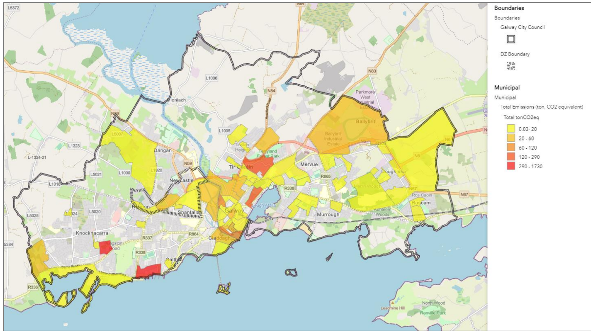
Fíor 4-5 Teasláráid déine astaíochtaí cathrach limistéar riaracháin Chomhairle Cathrach na Gaillimhe
